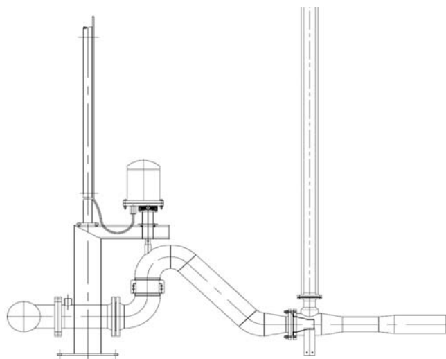
Schwenkeinheit der Reinigungseinrichtungen
